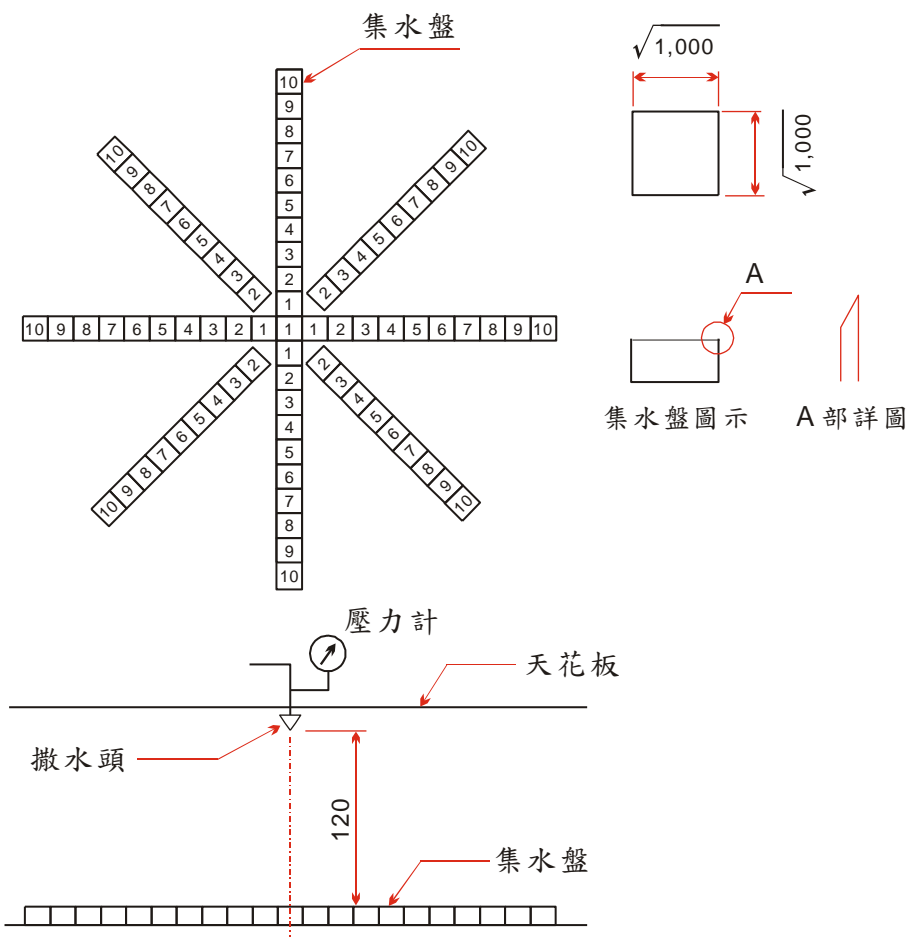
附圖 4 標準型、小區劃型及水道連結型撒水頭 撒水分布試驗裝置(單位：cm)
